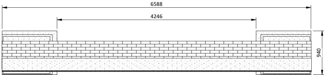
拱门-顶视图 1:50
