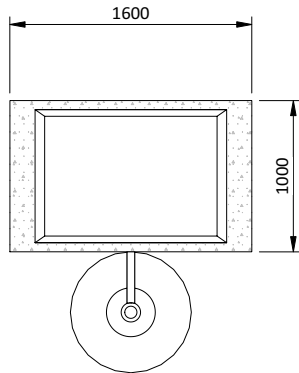
柱子-顶视图 1:50
