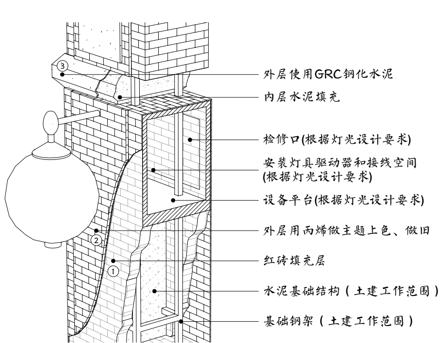
柱子结构解剖示意图
